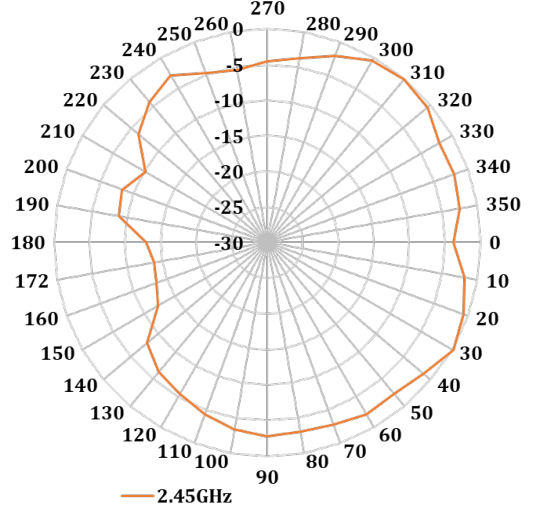
BLE antenna - Vertical
